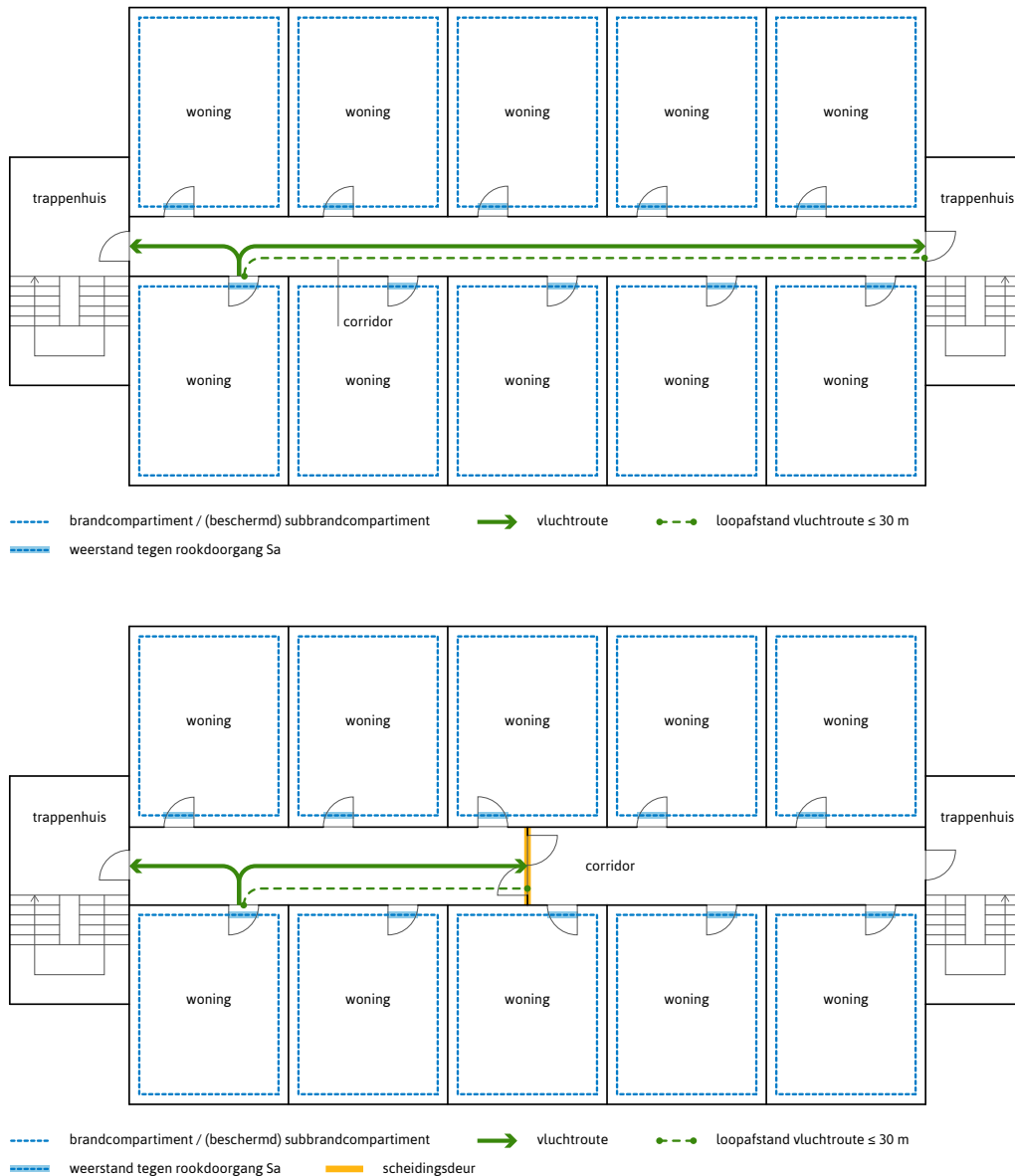
Figuur 3.2a en 3.2b: Woongebouw met corridor
