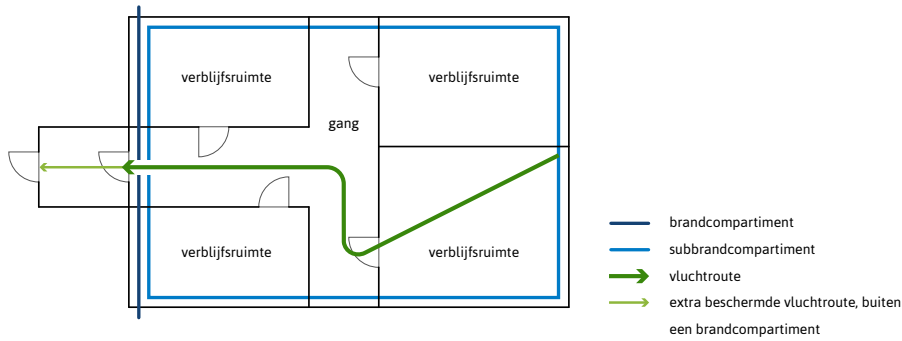
Figuur 2.3: Extra beschermde vluchtroute
