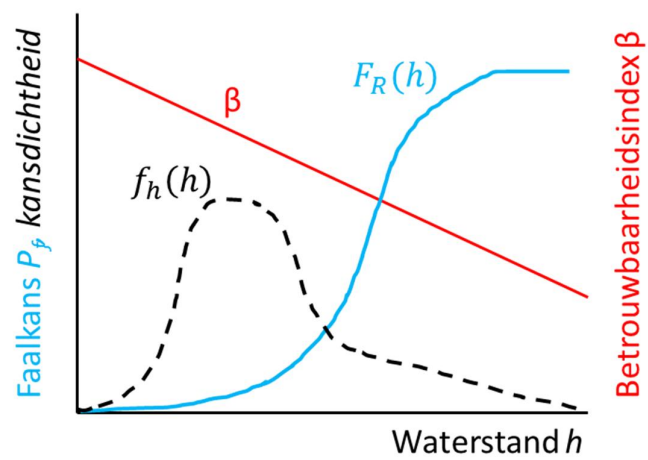
Figuur 6.2 Integreren fragility curve over kansdichtheid waterstand
