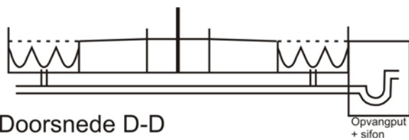
Figuur 11: Dwarsdoorsnede afdelingen met spoelsysteem en centrale afvoerleiding
